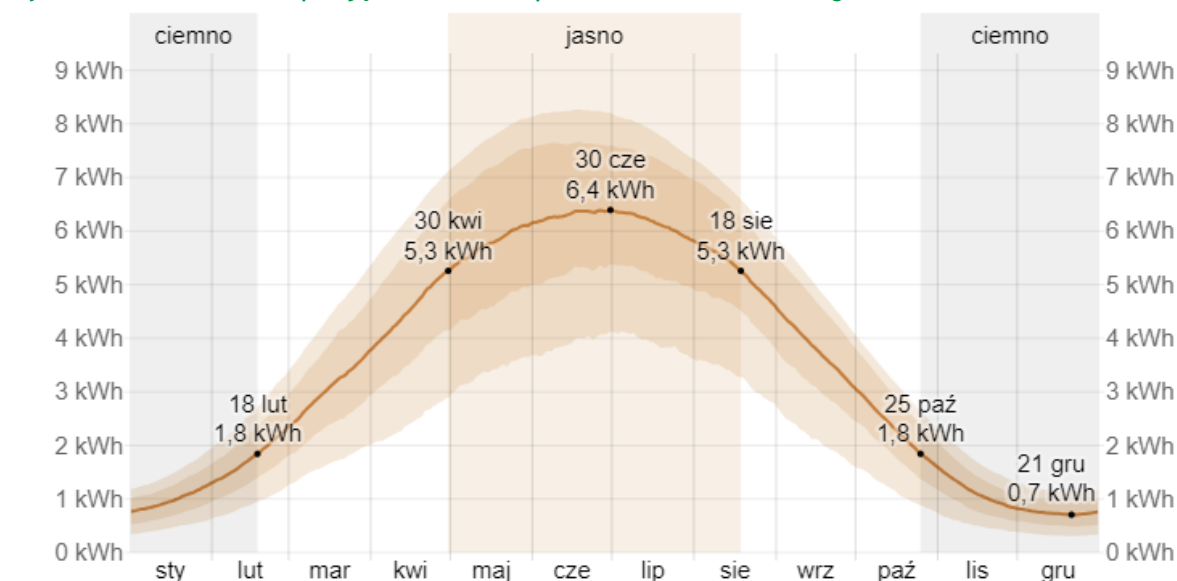
Wykres 27 - Średnie dobowe padające krótkofalowe promieniowanie słoneczne w gminie Jabłonna
